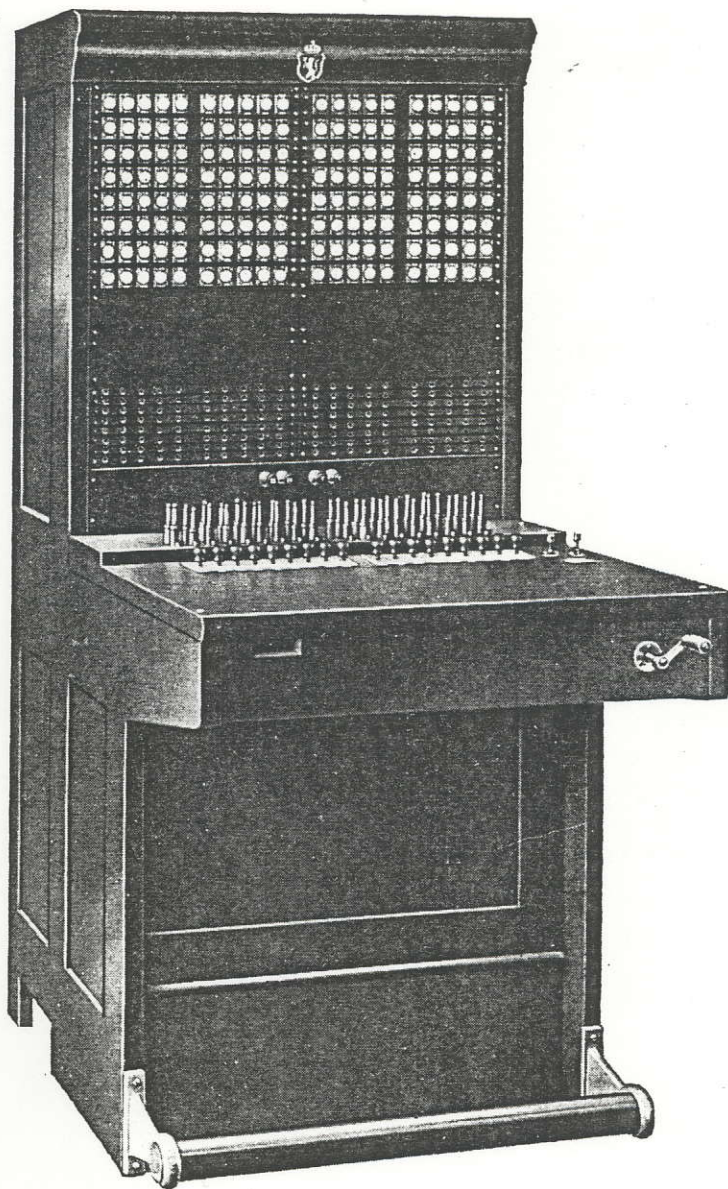
Snorvekslere. Kabinetype. Lokalbatterikobling. Klafsignaler.
