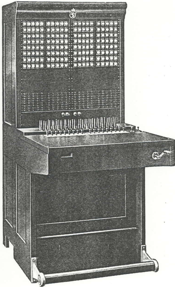
Snorvekslere. Kabinetttype. Centralbatterikobling. Klafsinaler.
