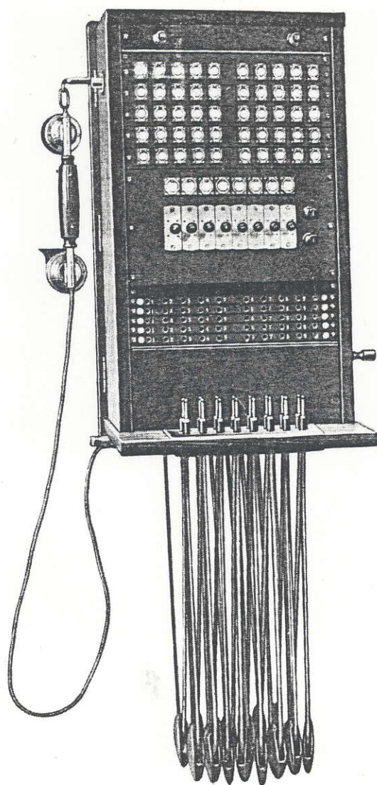
Snorvekslere med lokalbatterikobling for væg.
