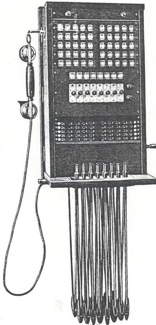
Snorvekslere for væg. Centralbatterikobling. Klafsignaler.
