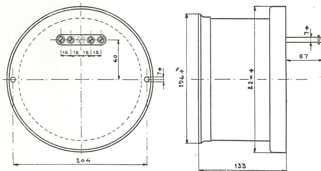
Wattmeter, type W 220 n og W 220.
