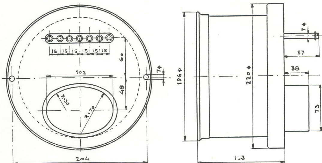
Wattmeter, type II W 220.
