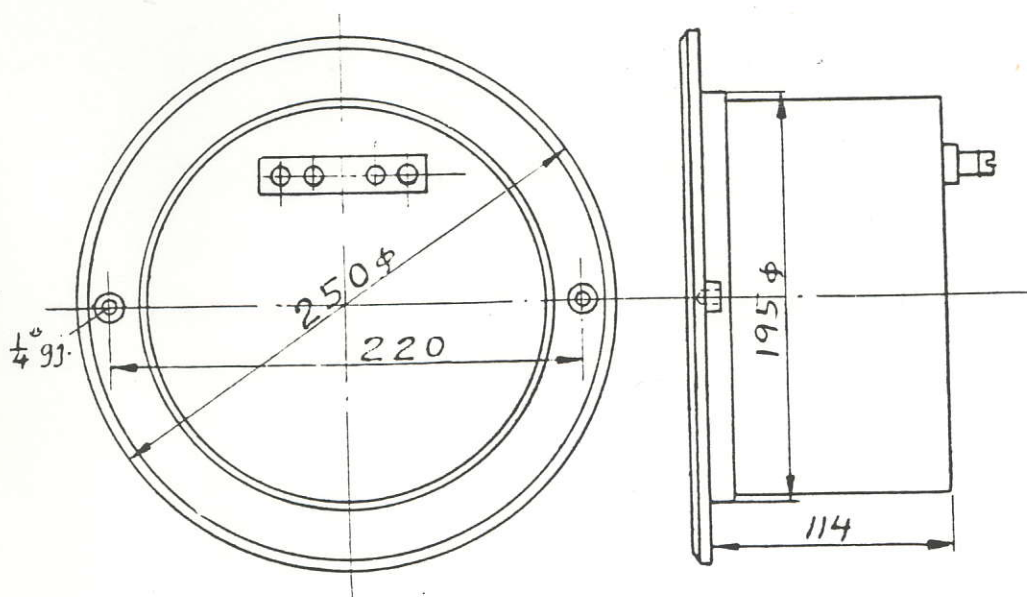
Wattmeter, type W 250 n og W 250.
